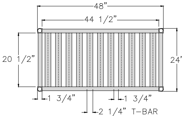
#2048TB Shelf
