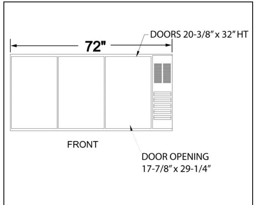
VBB-72
