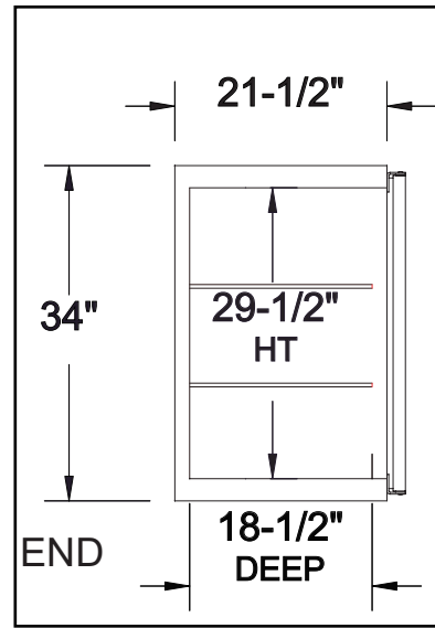
VBB-48 & VBB-72
